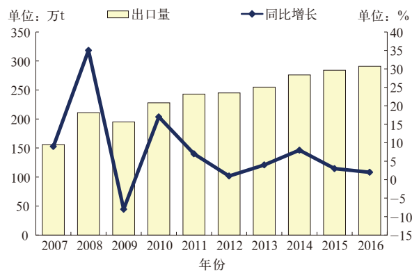
图34 2007—2016年纸制品出口情况
