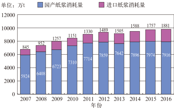
图18 2007—2016年纸浆总消耗情况
