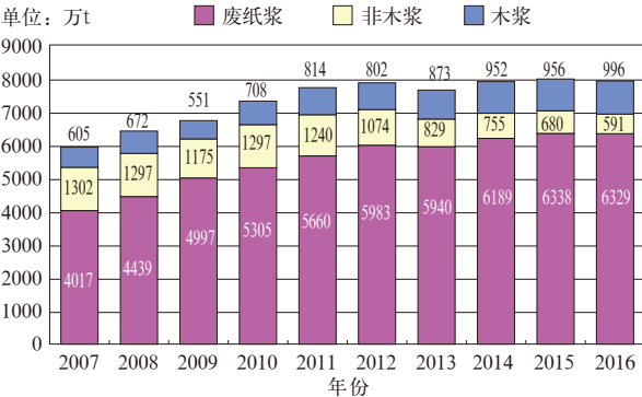
图17 2007—2016年国产纸浆消耗情况
